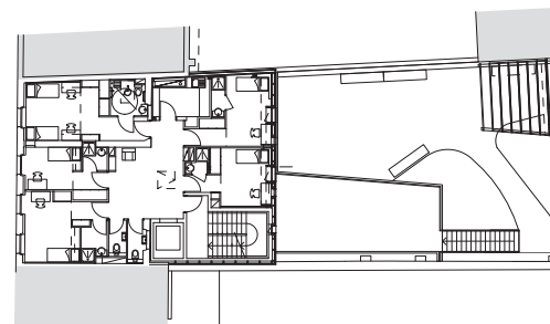
PLAN DES ÉTAGES DES CHAMBRES
