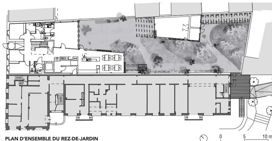
PLAN D'ENSEMBLE DU REZ-DE-JARDIN
